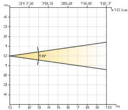
Standard Lens: 16°
