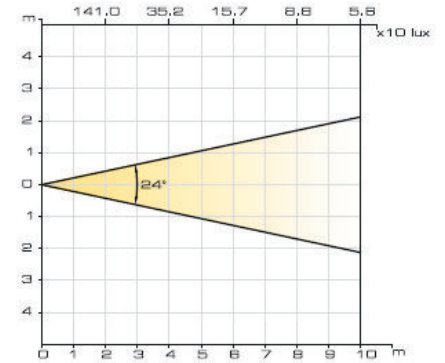
Lens: 24°
